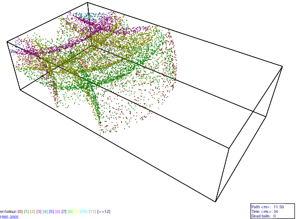
Abbildung 12 Berechnung der Schallausbreitung in einer Turnhalle nach dem Ray Tracing Verfahren (Geometrische Akustik). Hier sind 10000 Billardkugeln dargestellt, 34 Tausendstel Sekunden nach „Abschiessen“ bei der Schallquelle.
