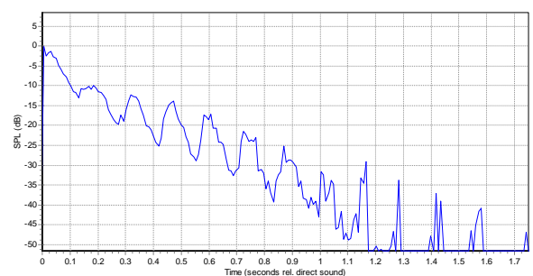
Abbildung 13 Berechnete Verlauf des Schallpegels in Funktion der Zeit für den in Abbildung 17 dargestellt. Situation. Es sind deutlich die periodisch wiederkehrenden Echos zu erkennen, welche als Flatterecho die Sprachverständlichkeit vermindern.
